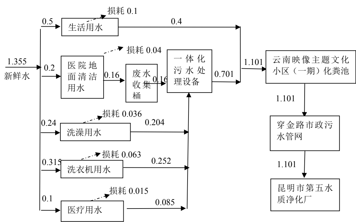
图 4-1 项目水平衡图 单位：m³/d
