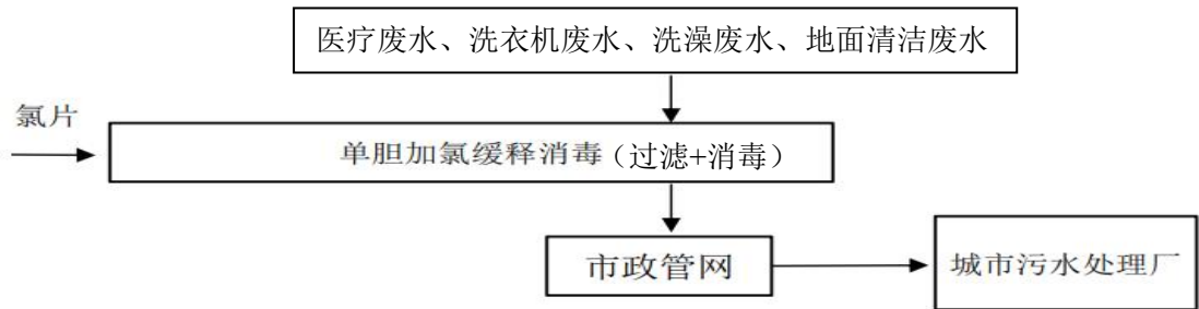
图 4-3 一体化污水处理设备工艺流程
