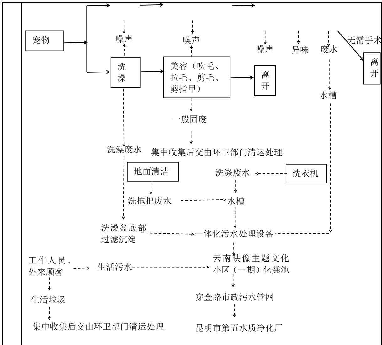
图 2-2 运营期工艺流程及产污节点图
