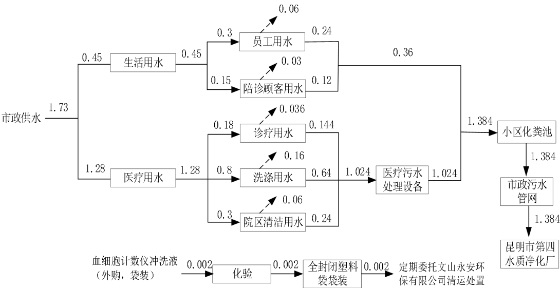
图 2-5 现有项目水平衡图 单位：m 3 /d
