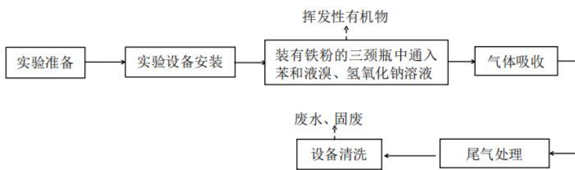
图 2-18 苯的溴代反应实验流程图
