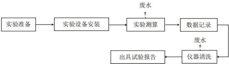
图 2-6 测算类物理实验流程图
