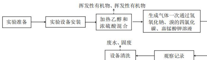
图 2-17 乙烯的制取实验流程图
