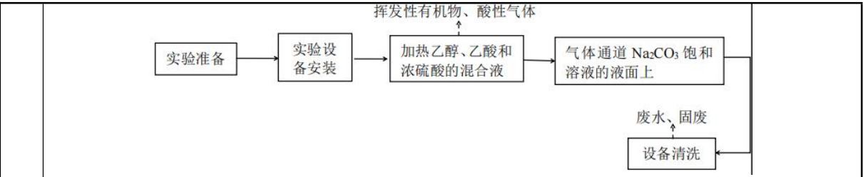
图 2-19 乙酸的酯化实验流程图
