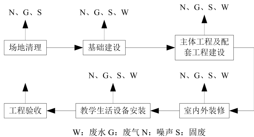
图 2-3 项目施工期产污流程图
