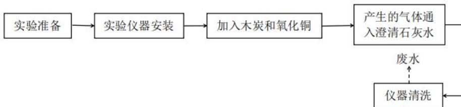
图 2-14 木炭还原氧化铜实验流程图
