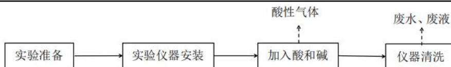
图 2-16 碱与酸反应实验流程图
