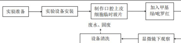
图 2-8 DNA 和 RNA 观察实验流程图
