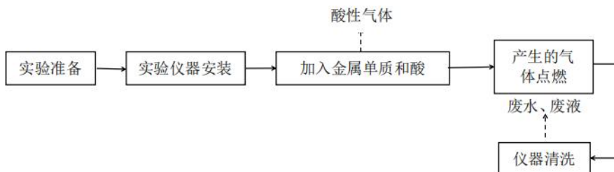
图 2-15 金属与酸反应实验流程图
