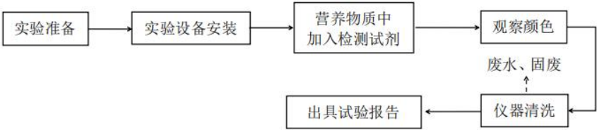
图 2-7 营养物质检测实验流程图
