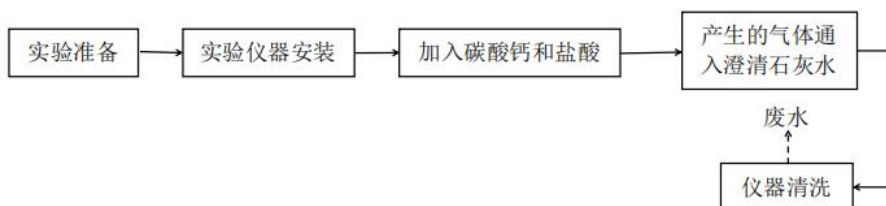
图 2-13 二氧化碳制备实验流程图
