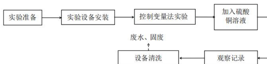
图 2-10 控制变量法研究酶的专一性和影响条件实验流程图
