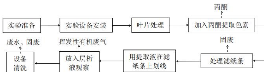
图 2-11 色素提取实验流程图
