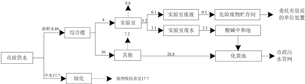
图 2-1 项目非雨天水平衡
