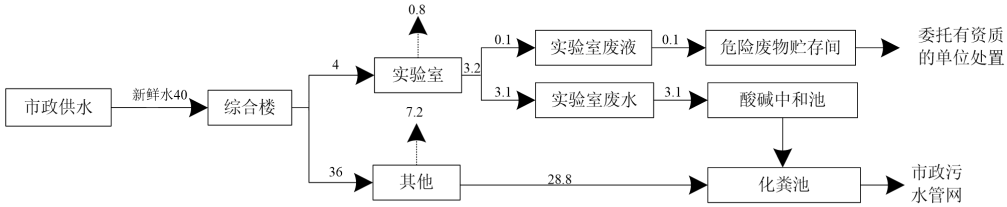
图 2-2 项目雨天水平衡
