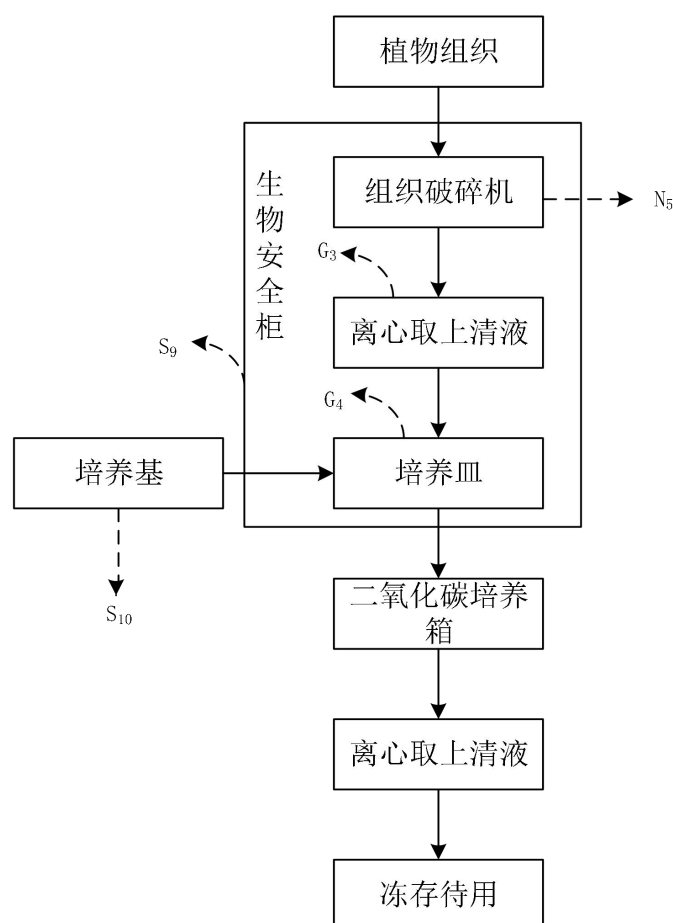
图 2-8 植物细胞培养工艺流程及产污节点图
