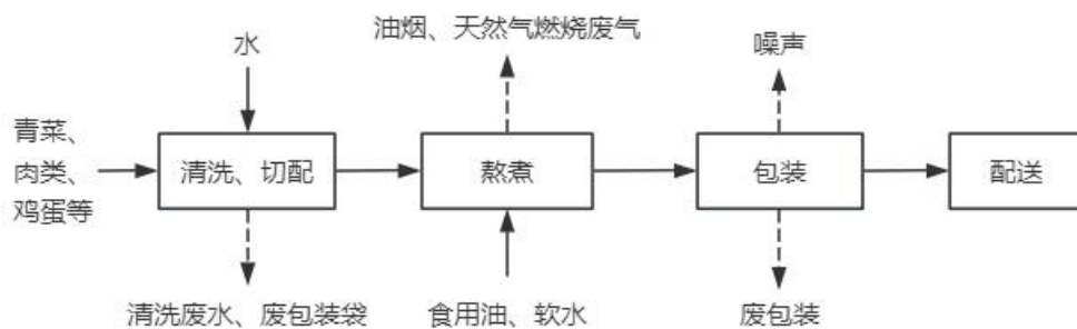
图 2-5 炒菜生产工艺流程图
