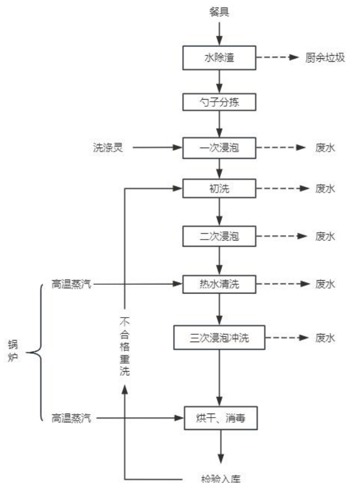
图 2-6 餐具清洗消毒工艺流程图及产污节点图
