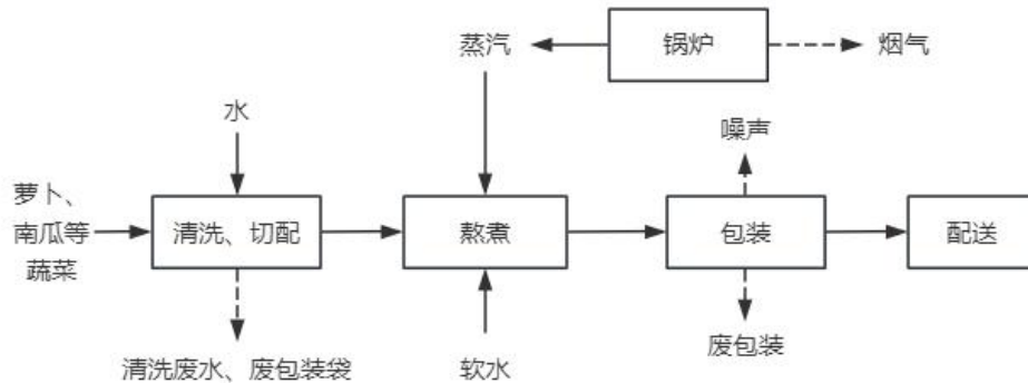
图 2-4 汤食生产工艺流程图
