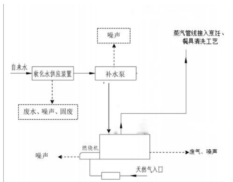
图 2-7 锅炉产生蒸汽和热空气产污环节示意图
