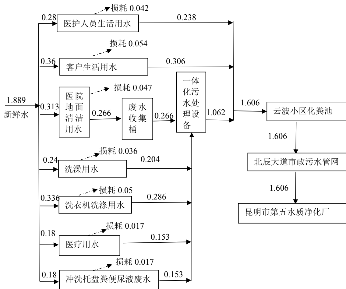
图 4-1 项目水平衡图 单位: \text{m}^3/\text{d}
