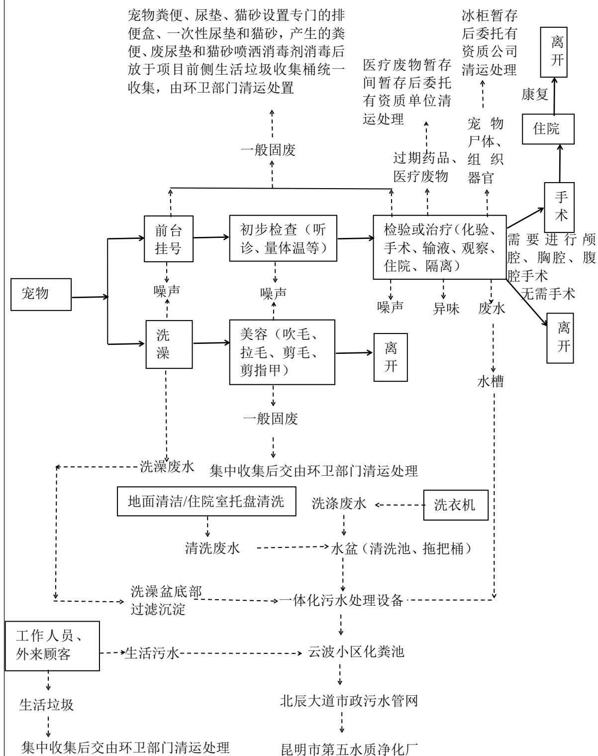
图 2-2 运营期工艺流程及产污节点图
