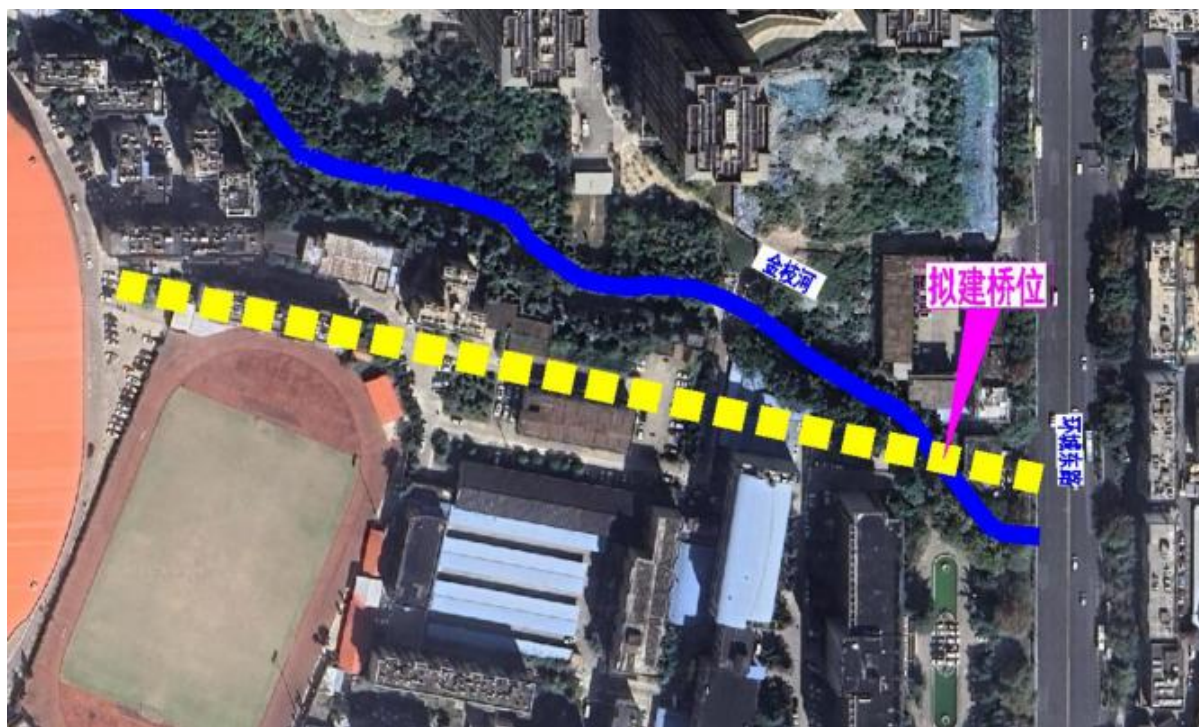
图 2-8 东通道桥梁建设位置
