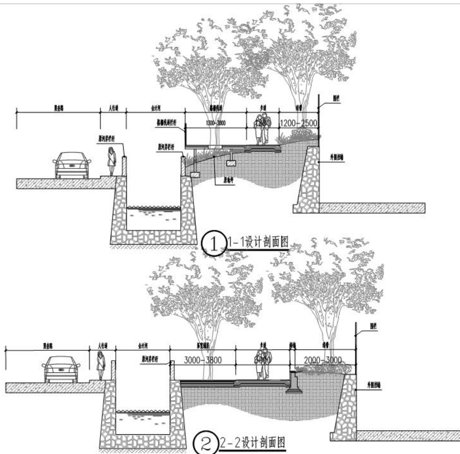
图 2-10 拓东路至状元楼段剖面图
