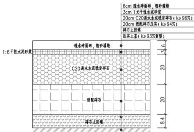
图 2-7 人行道路面结构图
