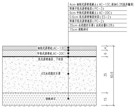
图 2-4 东通道工程路面结构图
