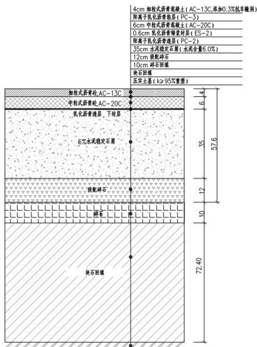
图 2-6 西通道工程路面结构图
