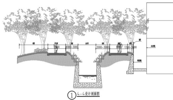
图 2-12 拓东体育场北门至环城北路段剖面图
