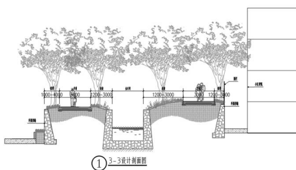
图 2-11 状元楼至拓东体育场北门段剖面图
