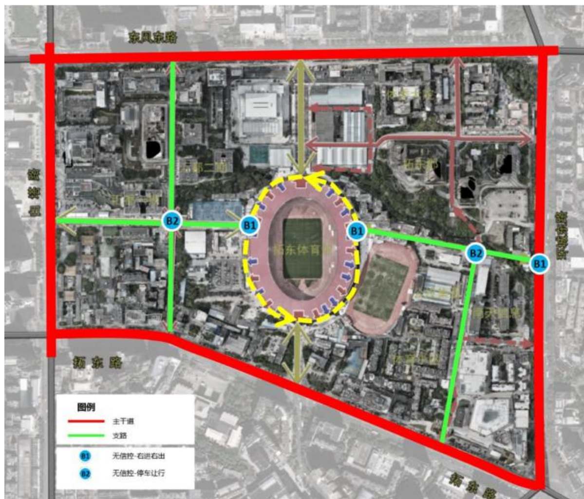
图 2-9 东西通道交叉口设置型式
