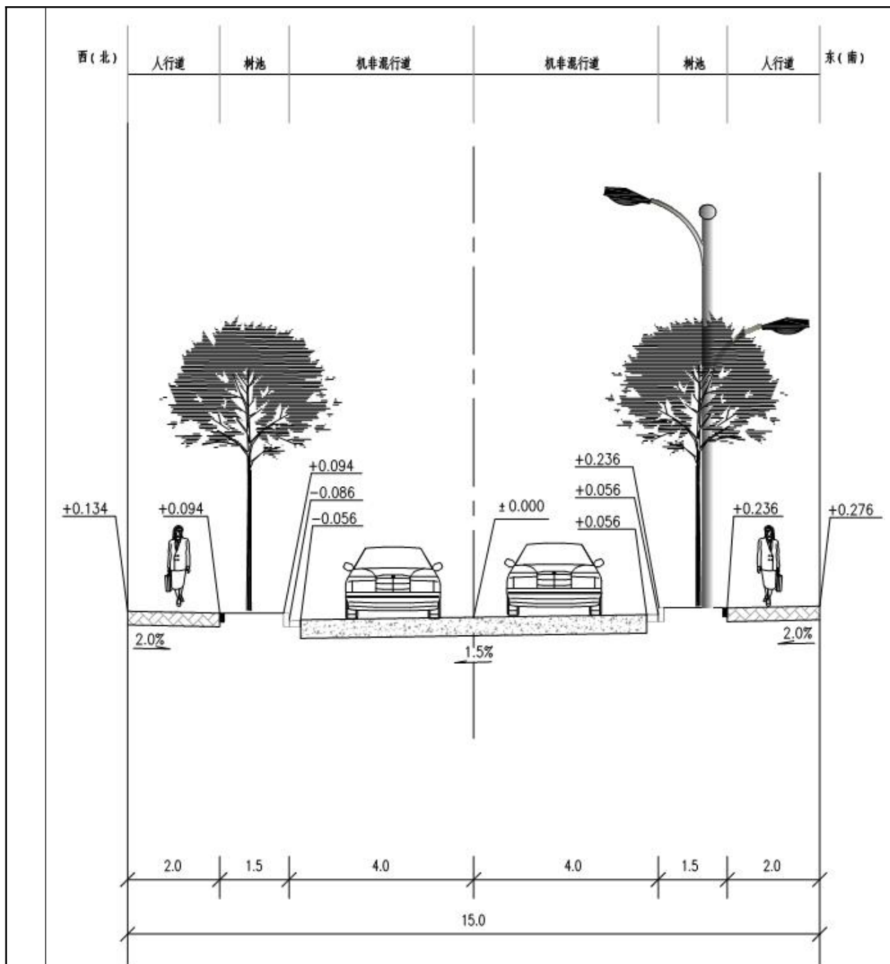
图 2-3 西通道 15m 标准横断面图
