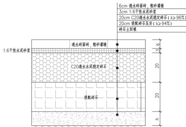
图 2-5 人行道路面结构图
